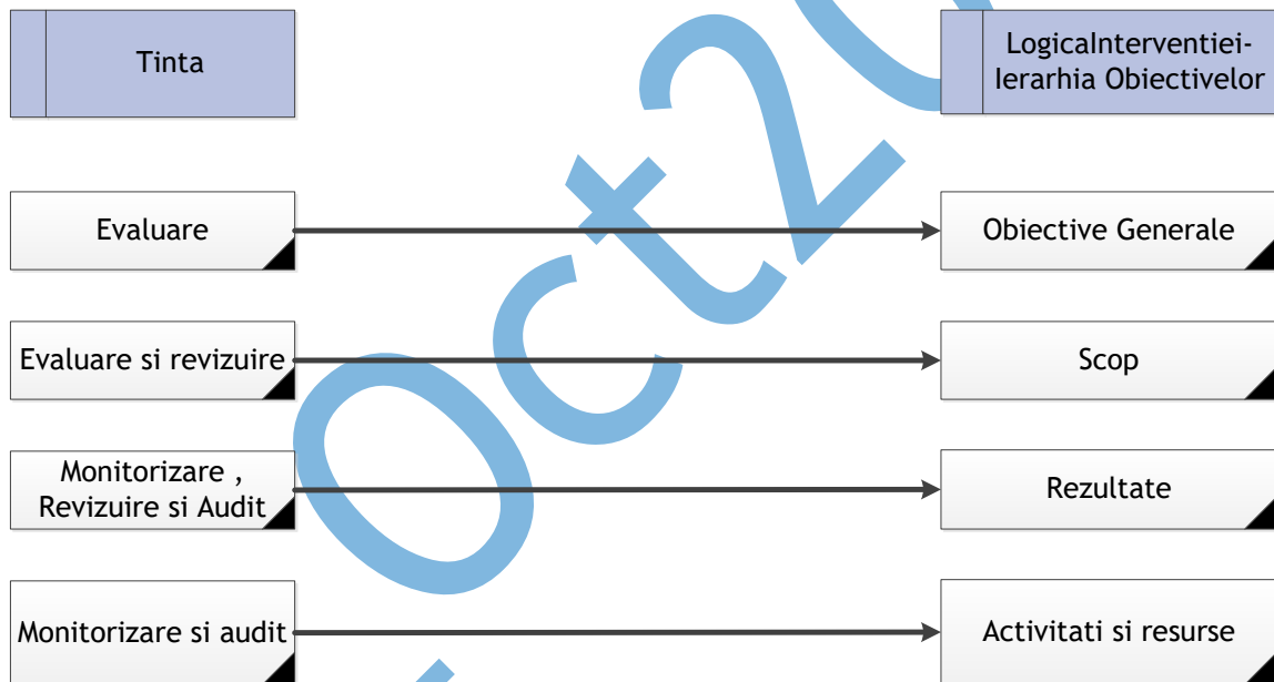
Figură 9. Monitorizare/Revizuire/Evaluare/Audit
